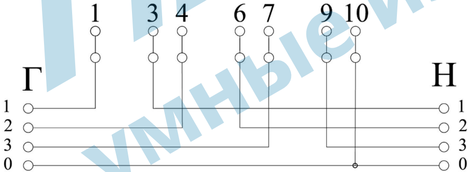
Схема включения счетчика
